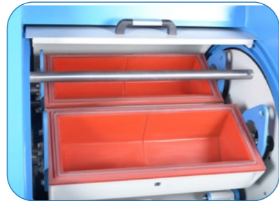
VKDT 140 Box Internal View VKDT 140 Kutu İç Görünümü
